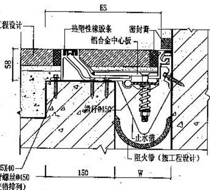
① 楼、地面与墙面 (SF-WS抗震型)
