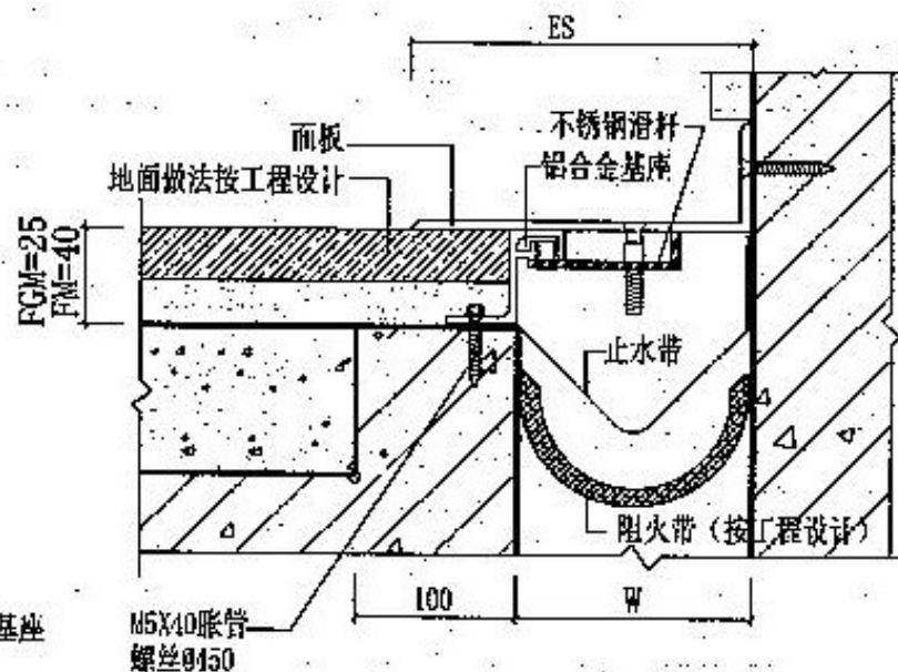
② 楼、地面与墙面 (F-WM/F-WGM金属盖板型)
