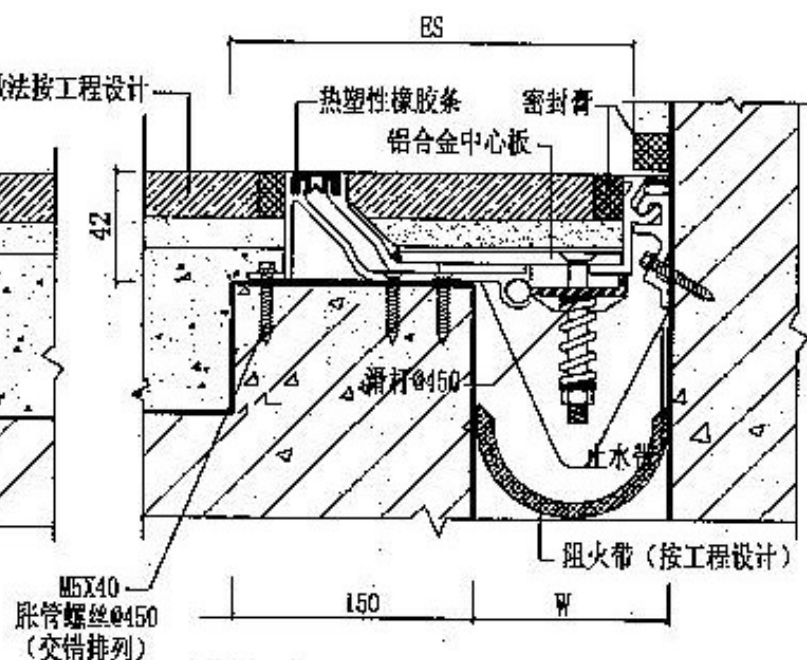
① 楼、地面与墙面 (SF-WES抗震型)
