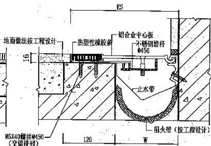
② 楼、地面 (F-WRWL双列嵌平型)
