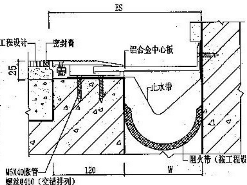
② 楼、地面与墙面 (F-WHL金属卡锁型)
