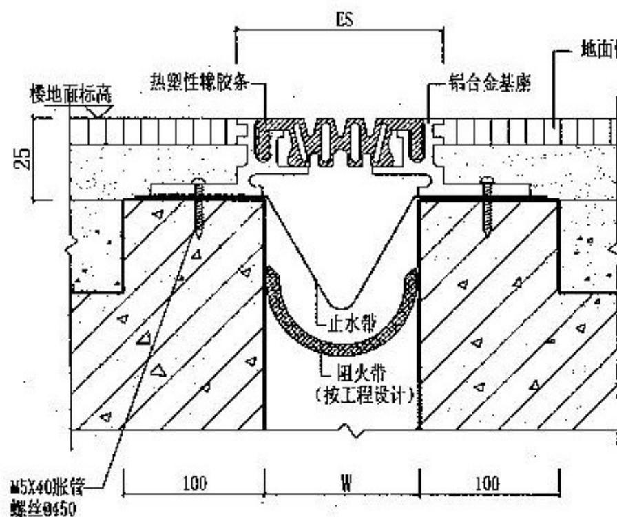
① 楼、地面 (FRG单列嵌平型)
