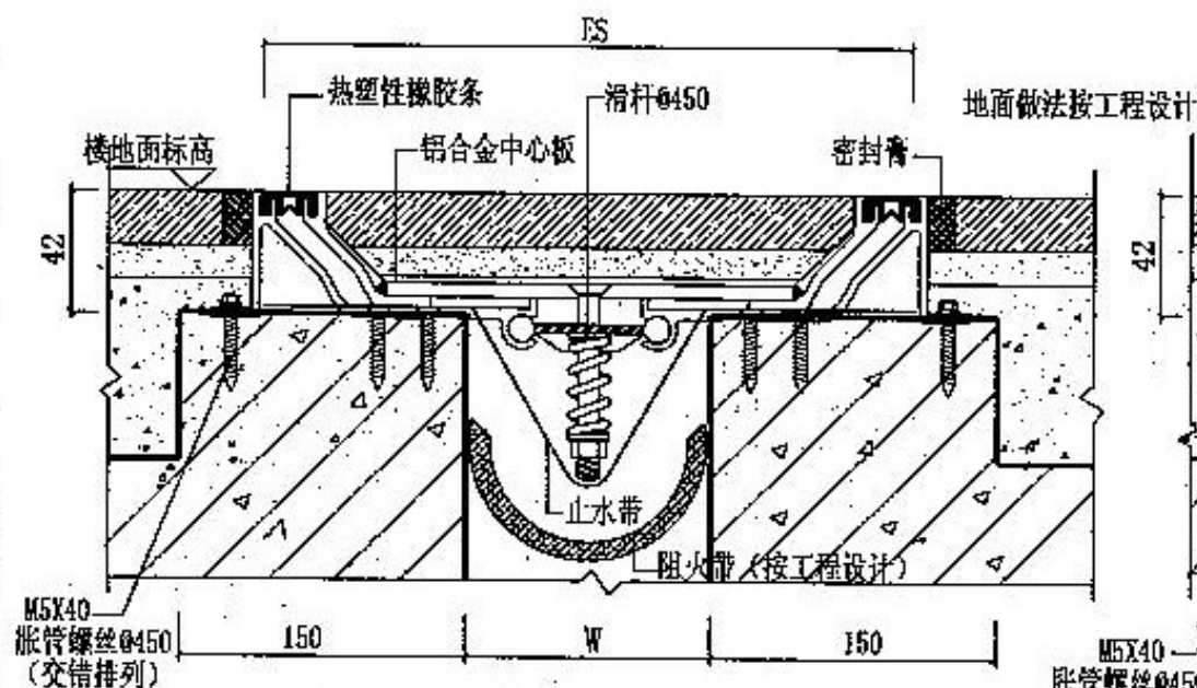
① 楼、地面 (SFES抗震型)
