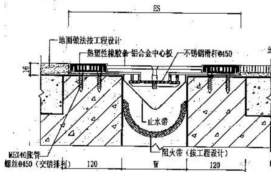
① 楼、地面 (FRWL双列嵌平型)
