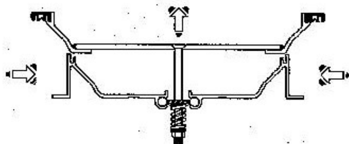
5. 中心板升起出边框, 可承受强烈地震时的位移
