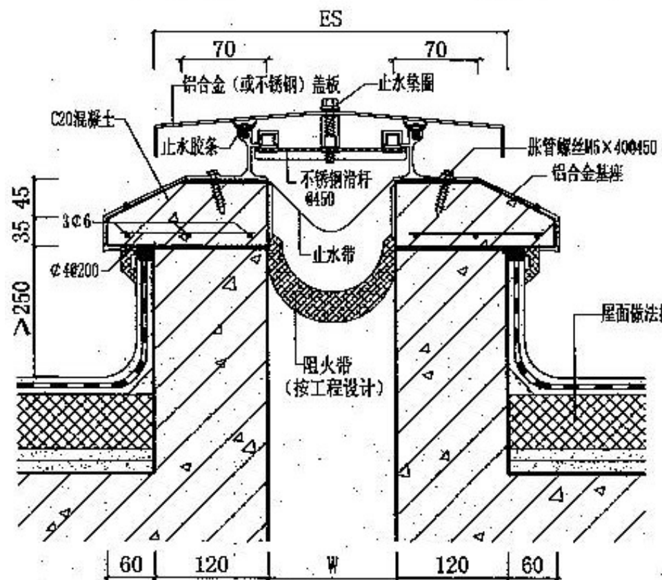
① 屋面变形缝 (RM金属盖板型)
