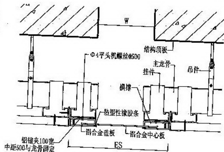
① 吊顶变形缝 (IL2金属卡锁型)
