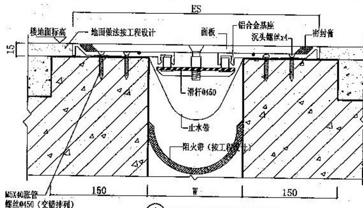
① 地面 (FDM金属盖板承重型)
