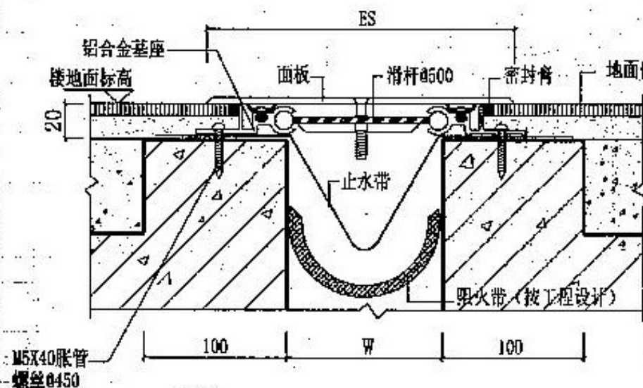
① 楼、地面 (FTM金属盖板型)
