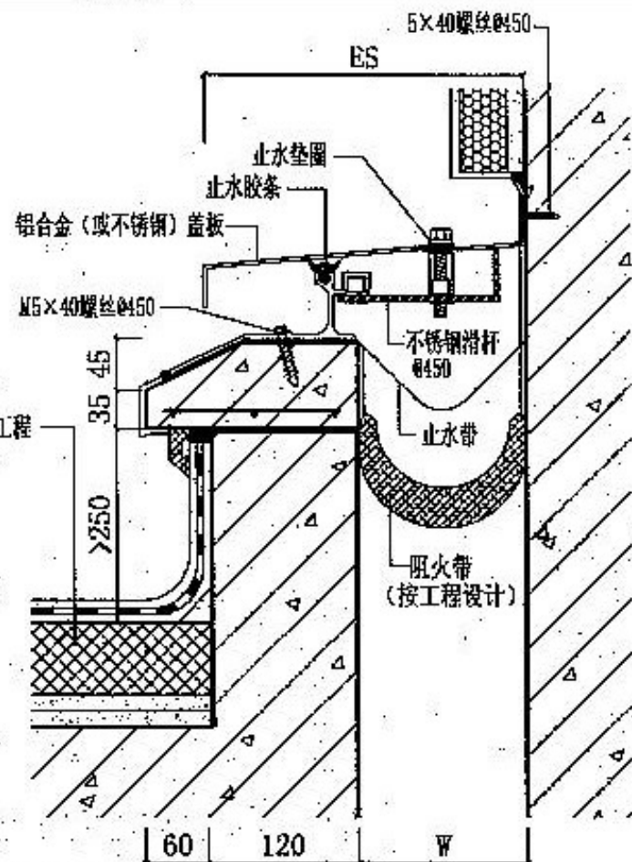
② 屋面变形缝 (R-WM金属盖板型)
