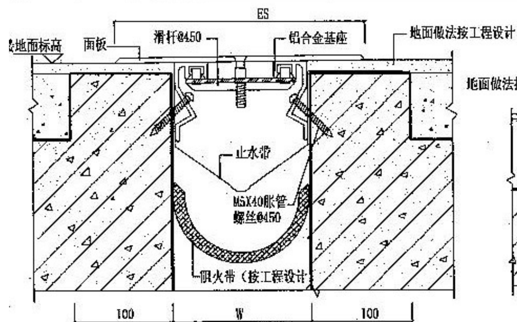
① 楼、地面 (FOM金属盖板型)
