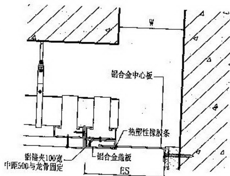
② 吊顶变形缝 (I-IL2金属卡锁型)
