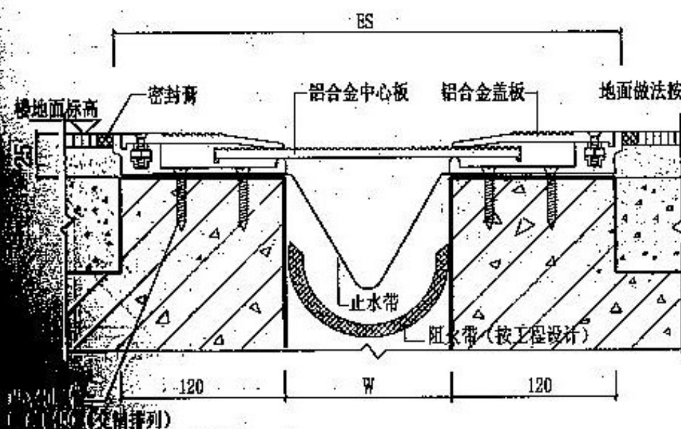
① 楼、地面 (FHL金属卡锁型)
